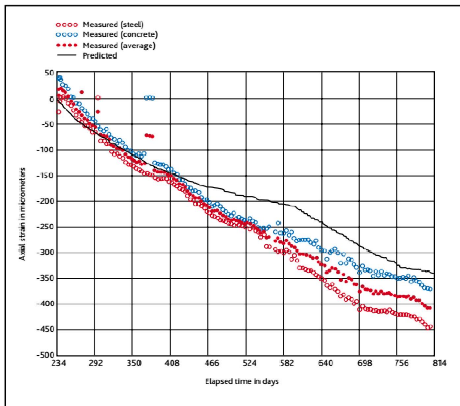
Hình 11.6 - So sánh các biến dạng dọc trực đo được và dự đoán của cột bê tông cốt thép trong nhà cao tầng trong quá trình xây dựng.
