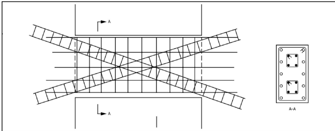
Hình 10.14 – Dầm cao nổi lỗ mở được cấu tạo cốt thép xiên.
