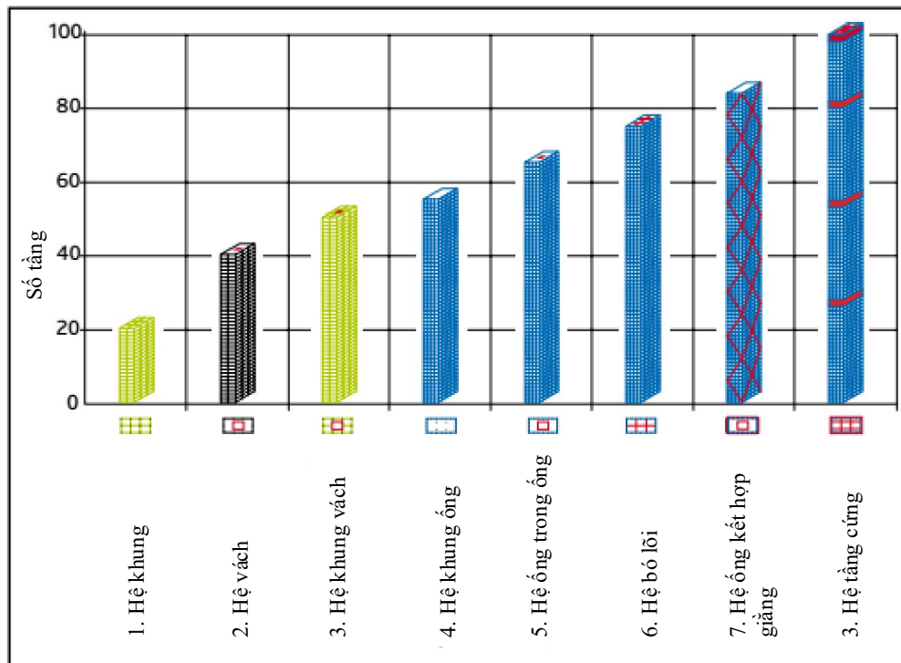
Hình 3.1 – Các hệ kết cấu chính
