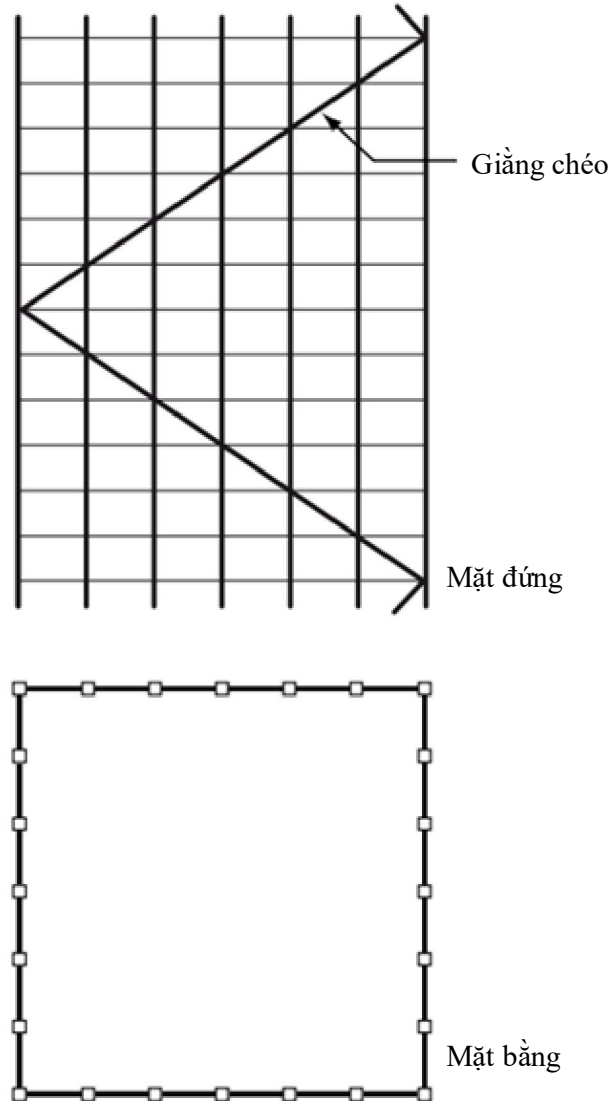
Hình 3.9 – Loại 7 – Hệ ống kết hợp giằng
