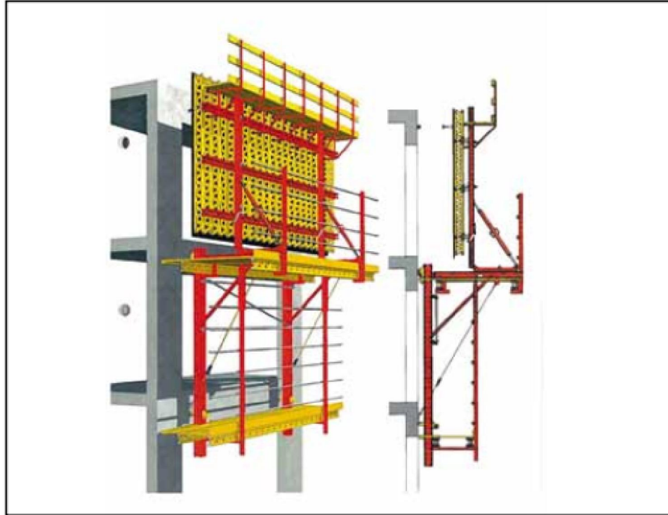
Figure 6.3 – Ví dụ về hệ ván khuôn nâng bằng cầu
