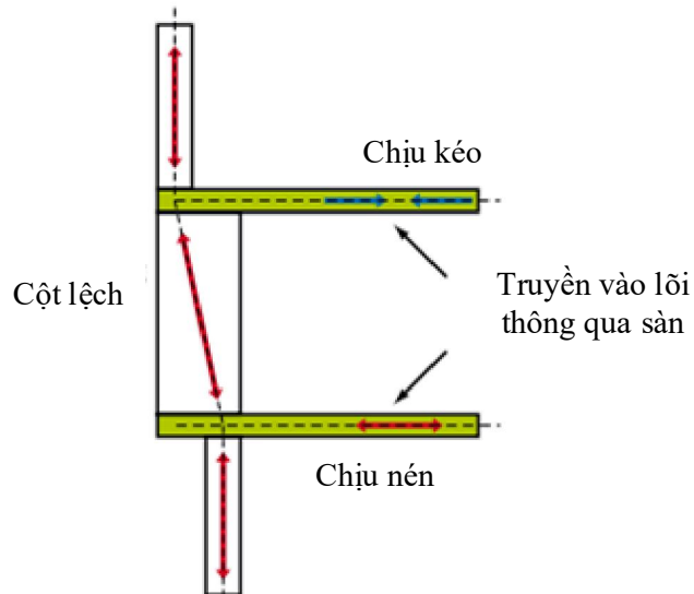
Hình 4.1 – Cột lệch
