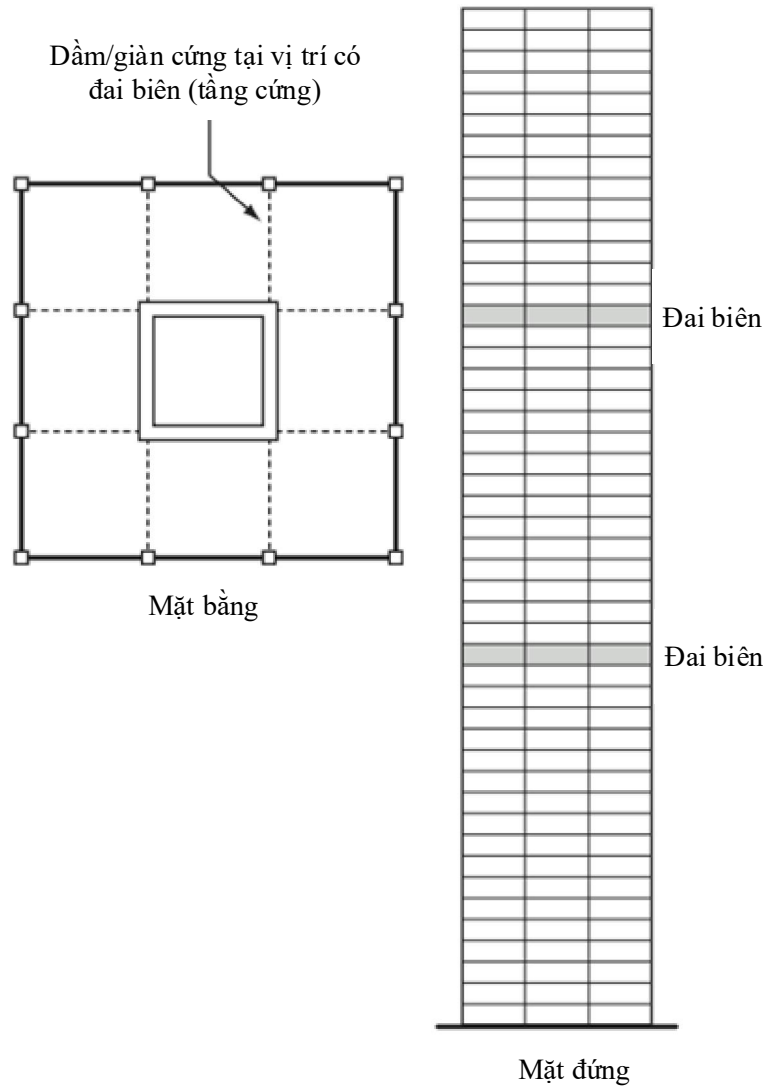
Hình 3.10 – Loại 8 – Hệ tầng cứng
