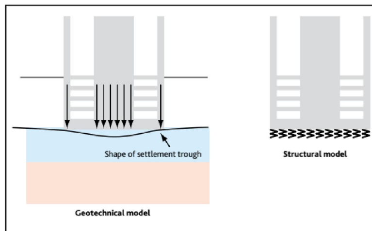
Hình 5.1 – So sánh mô hình phân tích địa kỹ thuật và mô hình kết cấu
