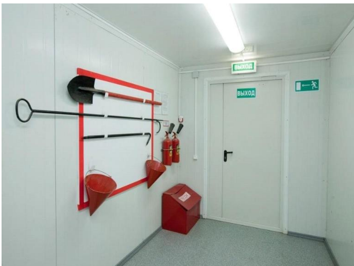
Hình 64 – Minh họa về bố trí các dụng cụ trong một phòng phương tiện chữa cháy ban đầu
