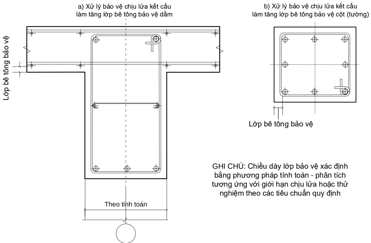
Hình 11 – Xử lý bảo vệ chịu lửa cho các kết cấu bê tông cốt thép bằng cách làm tầng lớp bê tông bảo vệ
