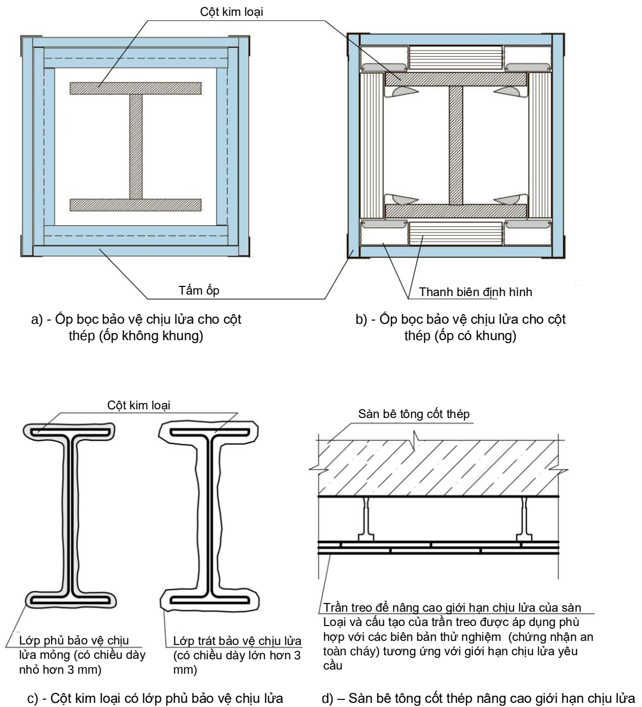
Hình 10 – Xử lý bảo vệ chịu lửa cho các dạng cấu kiện kết cấu cột, sàn
