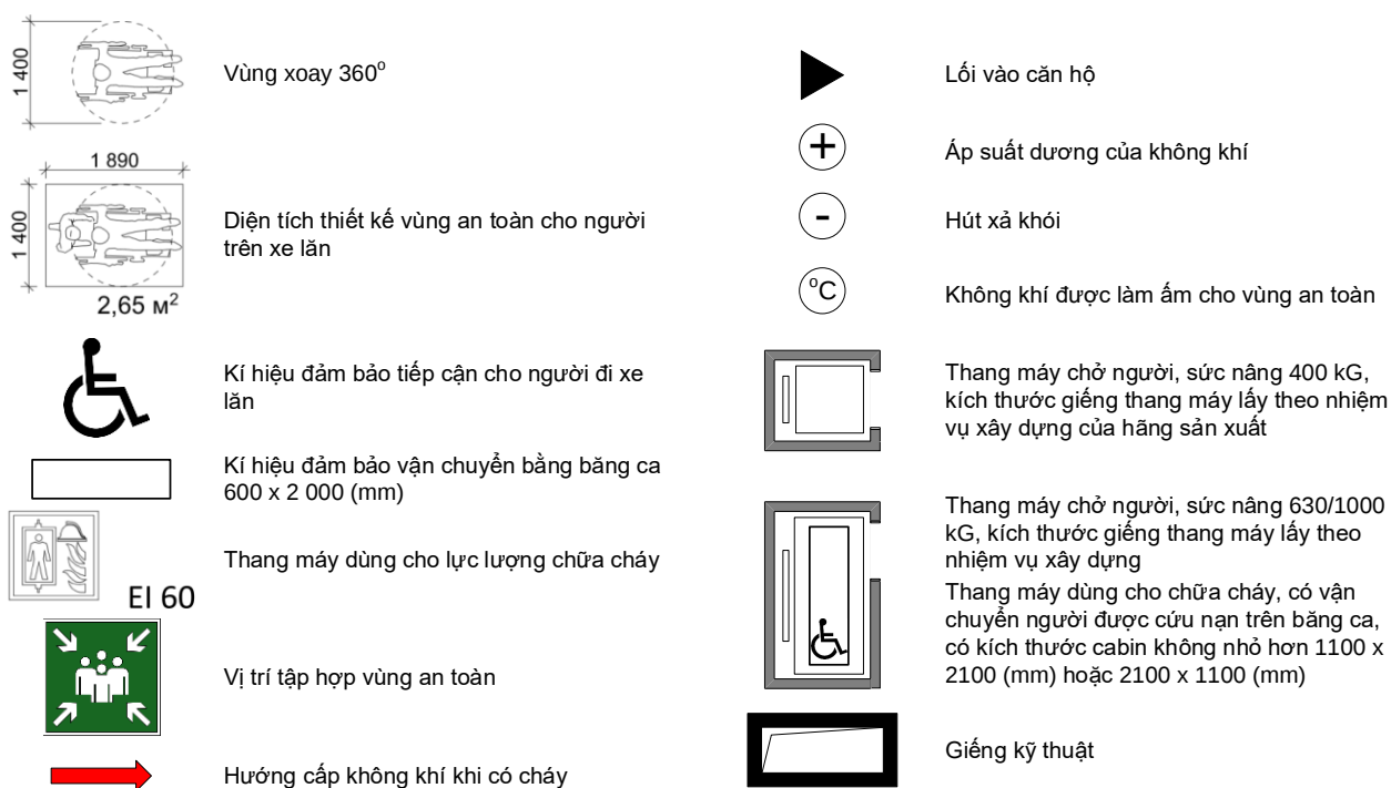
Hình 30 – Ký hiệu quy ước thể hiện trong các sơ đồ bố trí vùng an toàn ở các hình dưới đây
