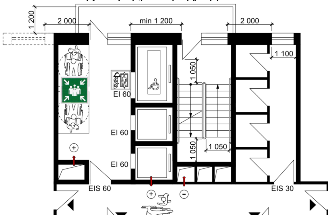
Hình 32 – Bố trí vùng an toàn trong sảnh thang máy chữa cháy bên cạnh buồng thang bộ loại N1
