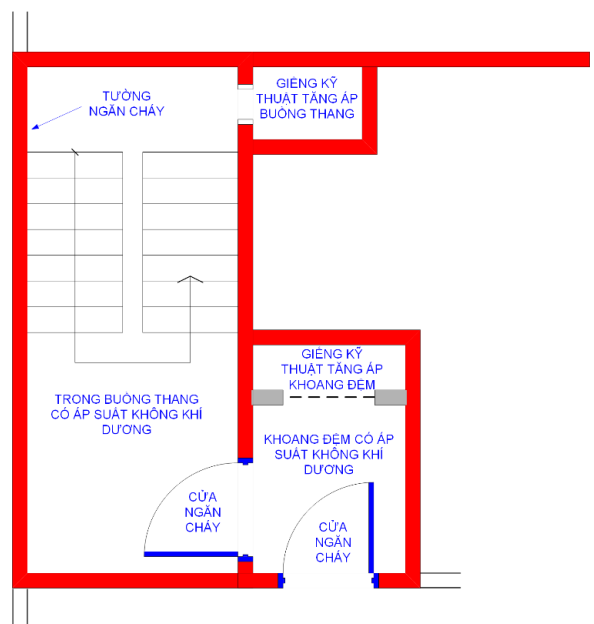
Hình 41 - Minh họa buồng thang bộ thoát nạn kết hợp N2 với N3 để thay thế giải pháp không nhiễm khói của buồng thang bộ N1
