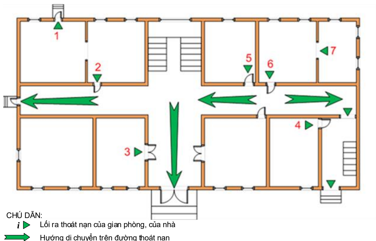
Hình 6 – Ví dụ minh họa về các lối ra thoát nạn của gian phòng và cửa nhà tại tầng có lối ra bên ngoài (tầng 1)
