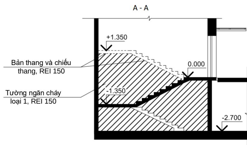
Hình 46 – Bố trí lối ra thoát nạn từ tầng hầm (gara ô tô) trực tiếp ra ngoài, tách riêng khỏi buồng thang bộ của phần trên (loại buồng thang bộ N1)
