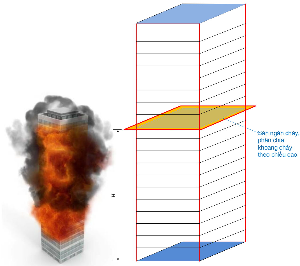
Hình 20 – Ví dụ về việc ngăn tách khoang cháy theo chiều cao để hạn chế quy mô đám cháy trong nhà chỉ sử dụng cho một công năng
