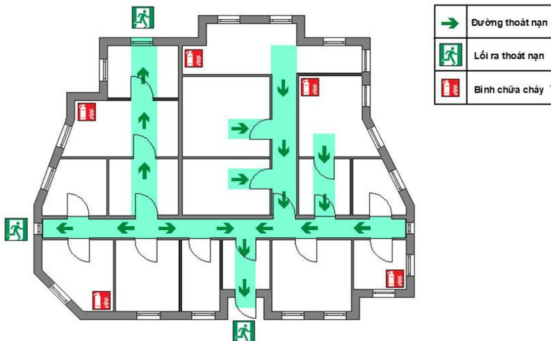
Hình 63 - Ví dụ về niêm yết sơ đồ thể hiện bố trí các lối ra thoát nạn và phương tiện chữa cháy ban đầu cho nhà
