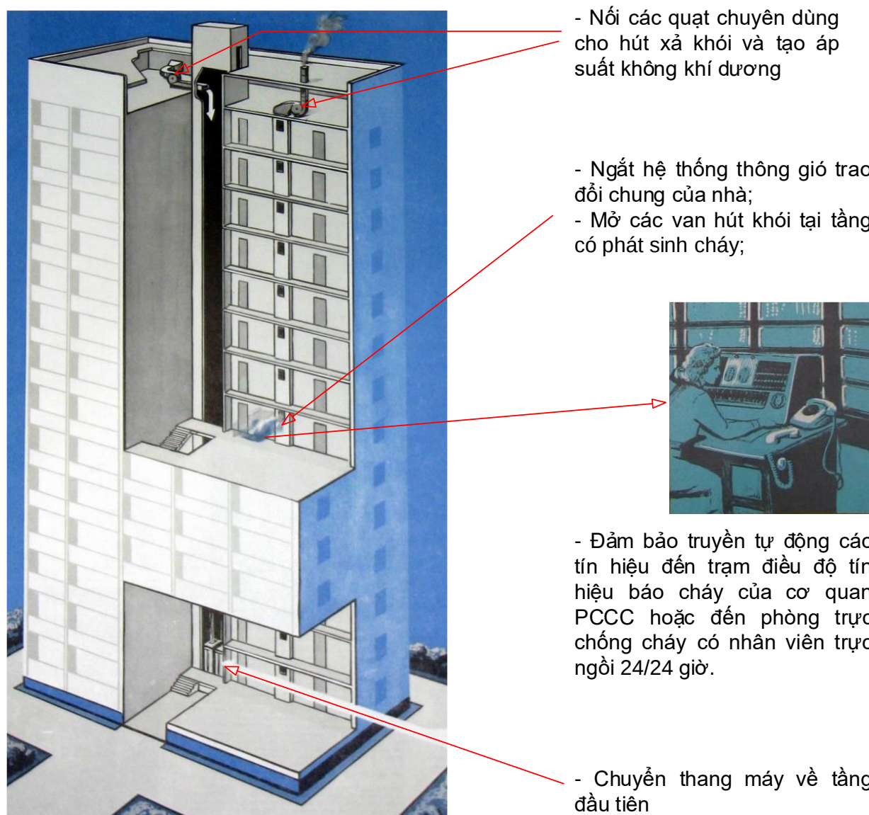
Hình 59 – Minh họa về các yêu cầu cơ bản đối với hệ thống bảo vệ chống khói của nhà cao trên 30 m
