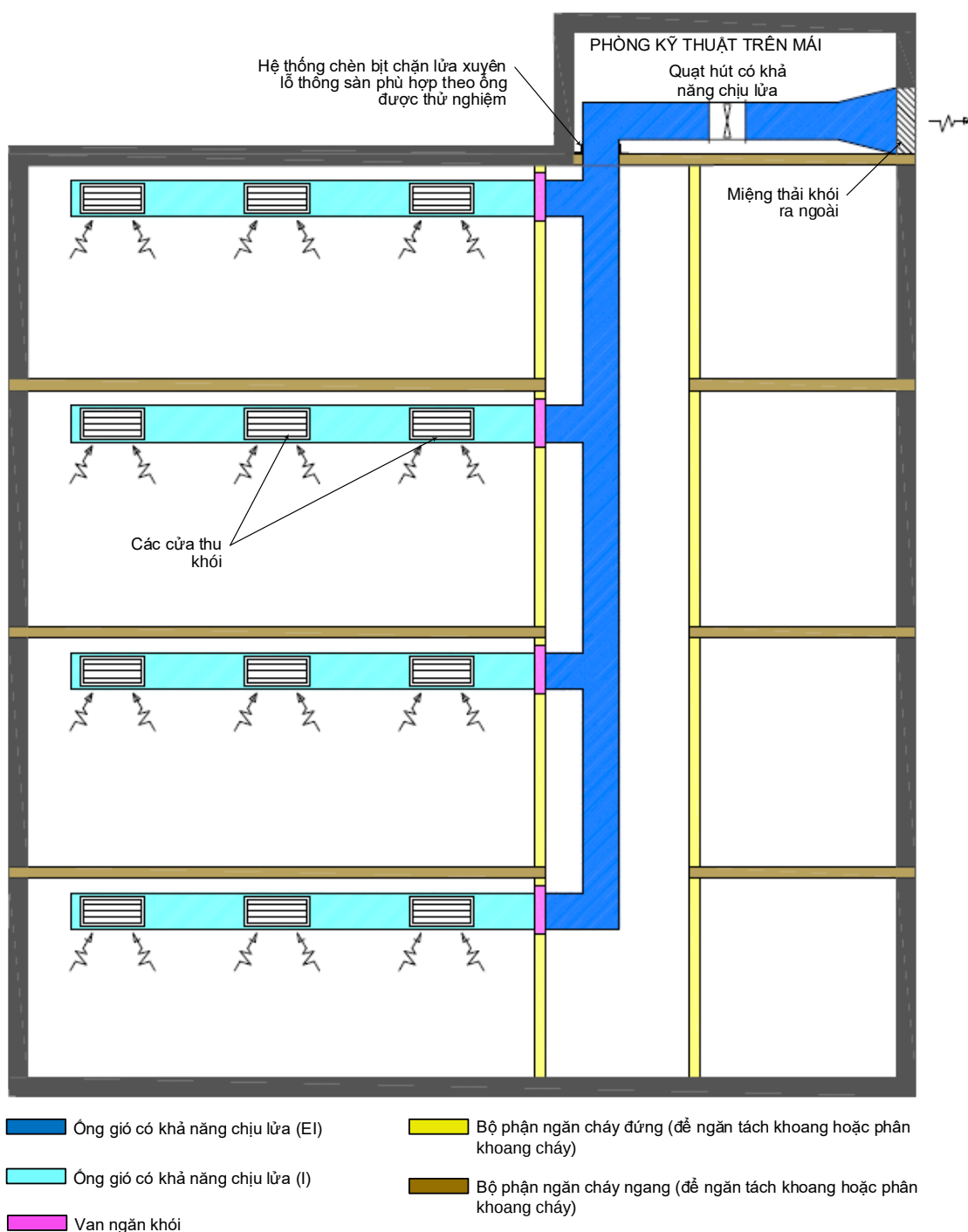
Hình 15 – Ví dụ về một hệ thống hút xả khói cho các tầng khác nhau
