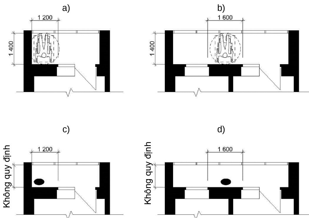
Hình 35 – Bố trí vùng an toàn bên cạnh lối ra khẩn cấp ở ban công và logia
