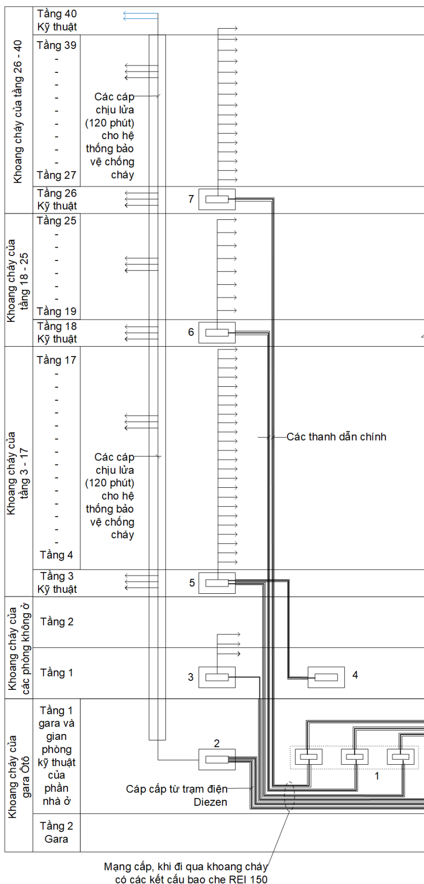
Hình 60 – Sơ đồ nguyên lý (cấu trúc) đặt mạng lưới điện 380/220 V (mặt cắt đứng) cho nhà cao tầng
