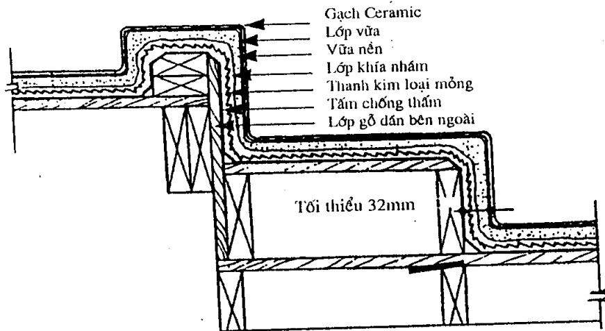
DẠNG KHUNG GỖ
