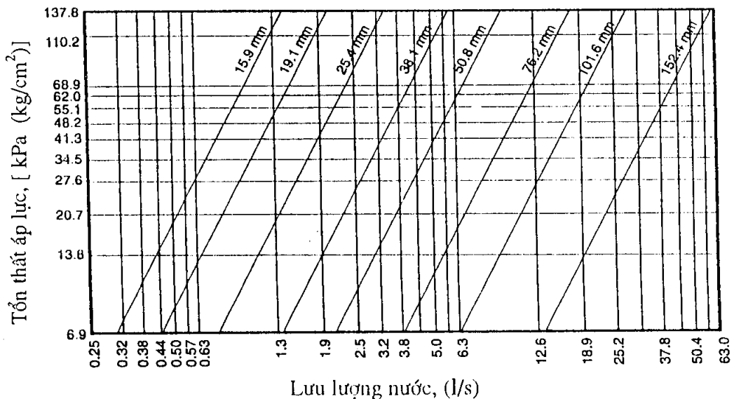
Tổn thất do ma sát của đồng hồ đo nước dạng đĩa
